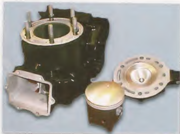
Cabeza de fuerza de motor de dos tiempos
